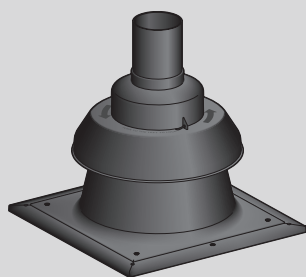
Płyta kominowa z ustnikiem
